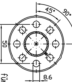
Befestigungsbohrungen
